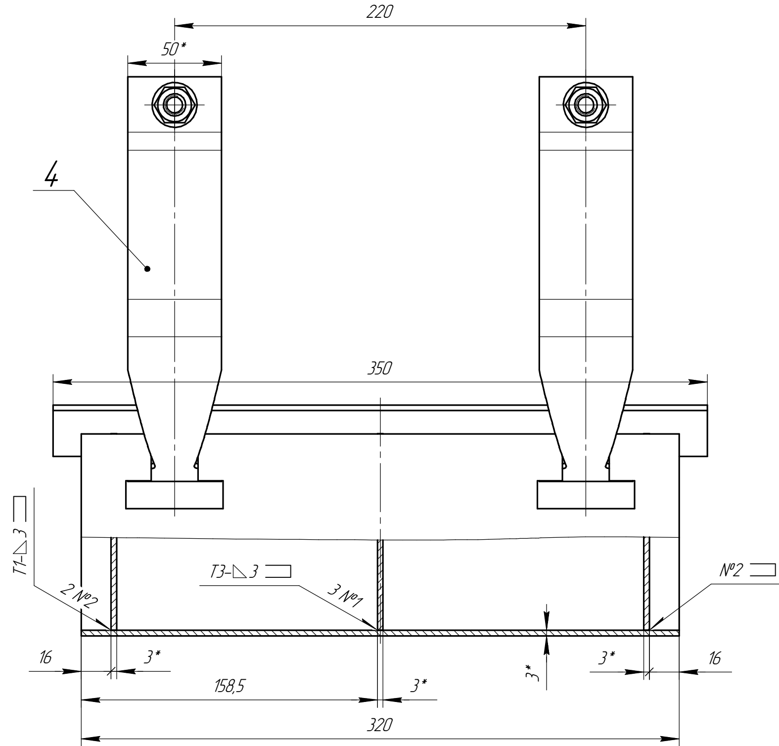
Дет. поз. 1 (1:4)
