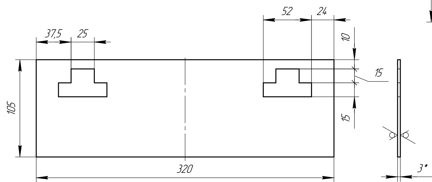
Дет. поз. 2 (1:2,5)
