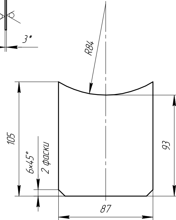
Дет. поз. 3
